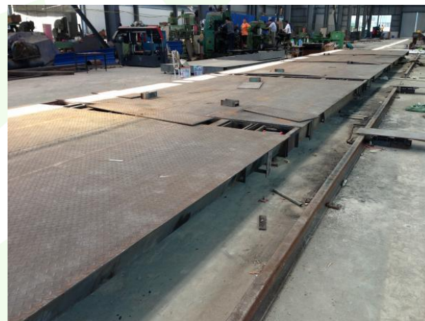
電子汽車稱重裝置
